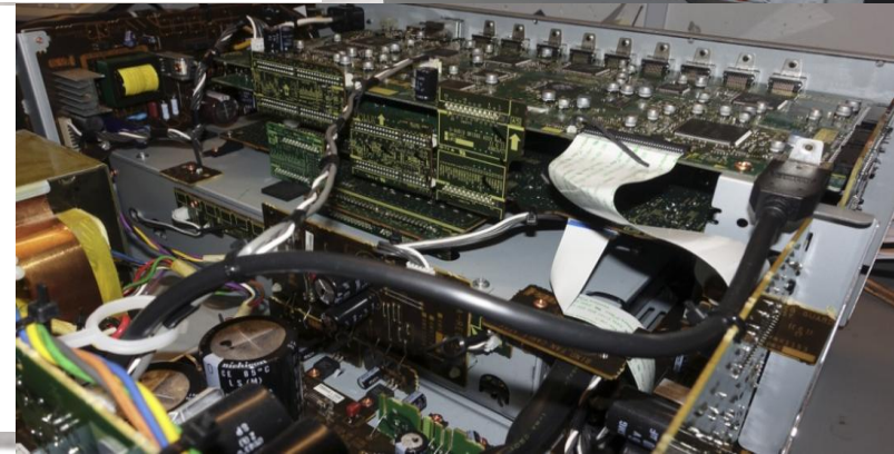
Separates abgeteiltes Gehäuse für Endstufen mit Lüfter
