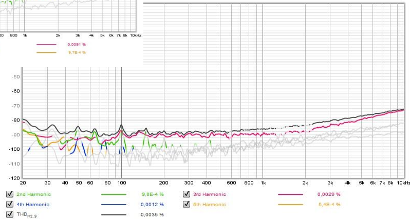
9V @ 32ohm
