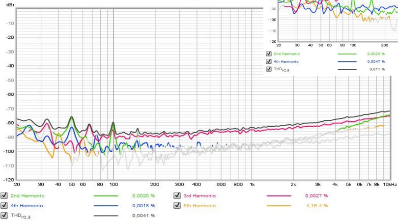
9V @ 4ohm
