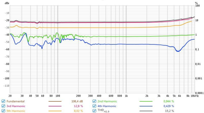
U70max, 4 ohm
