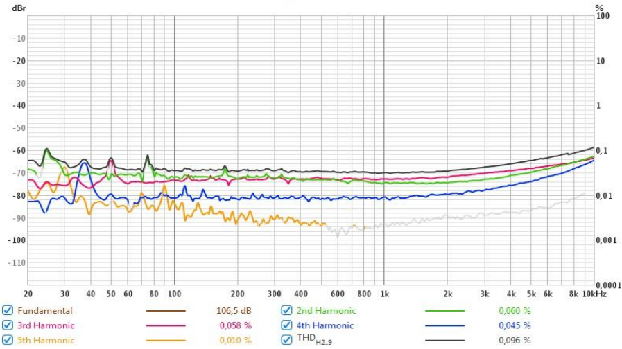
9V, 4 ohm
