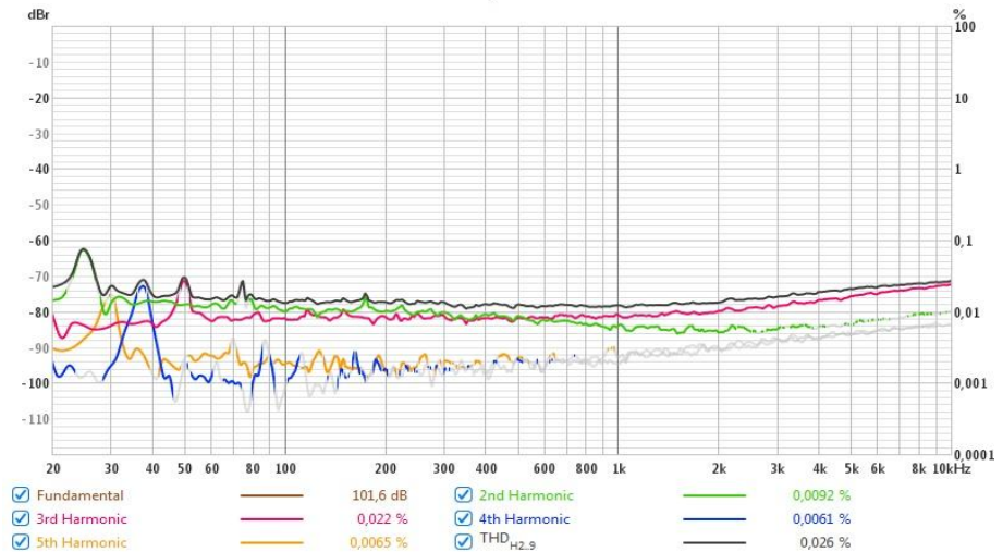
U70max, 32 ohm
