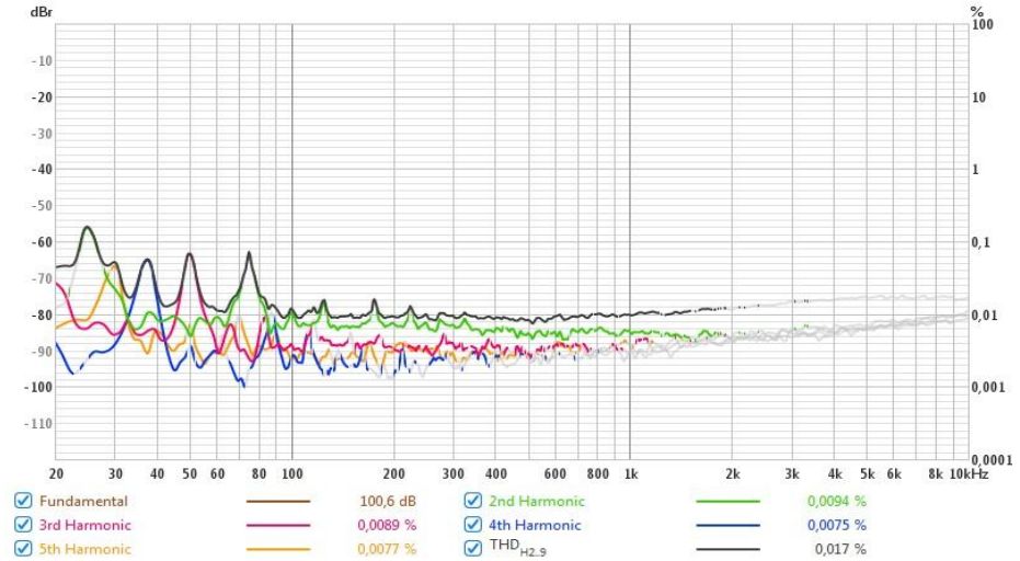
9V, 32 ohm
